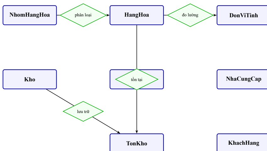
Hình 7.1: Sơ đồ ERD – Danh mục (Master Data)
