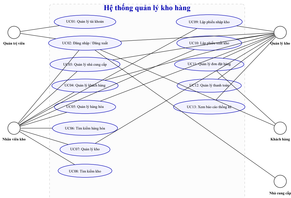
Hình 3.4: Sơ đồ use case tổng quát của hệ thống quản lý kho hàng
