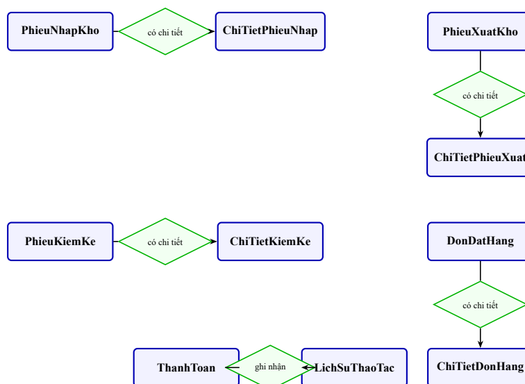
Hình 7.2: Sơ đồ ERD – Nghiệp vụ (Transaction)
